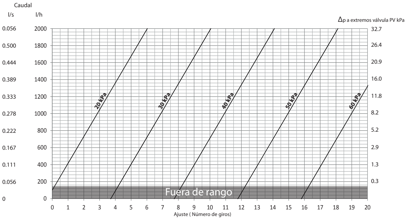
Gráfica de caudales Frese PV Compact DN 20, 20-60 kPa
