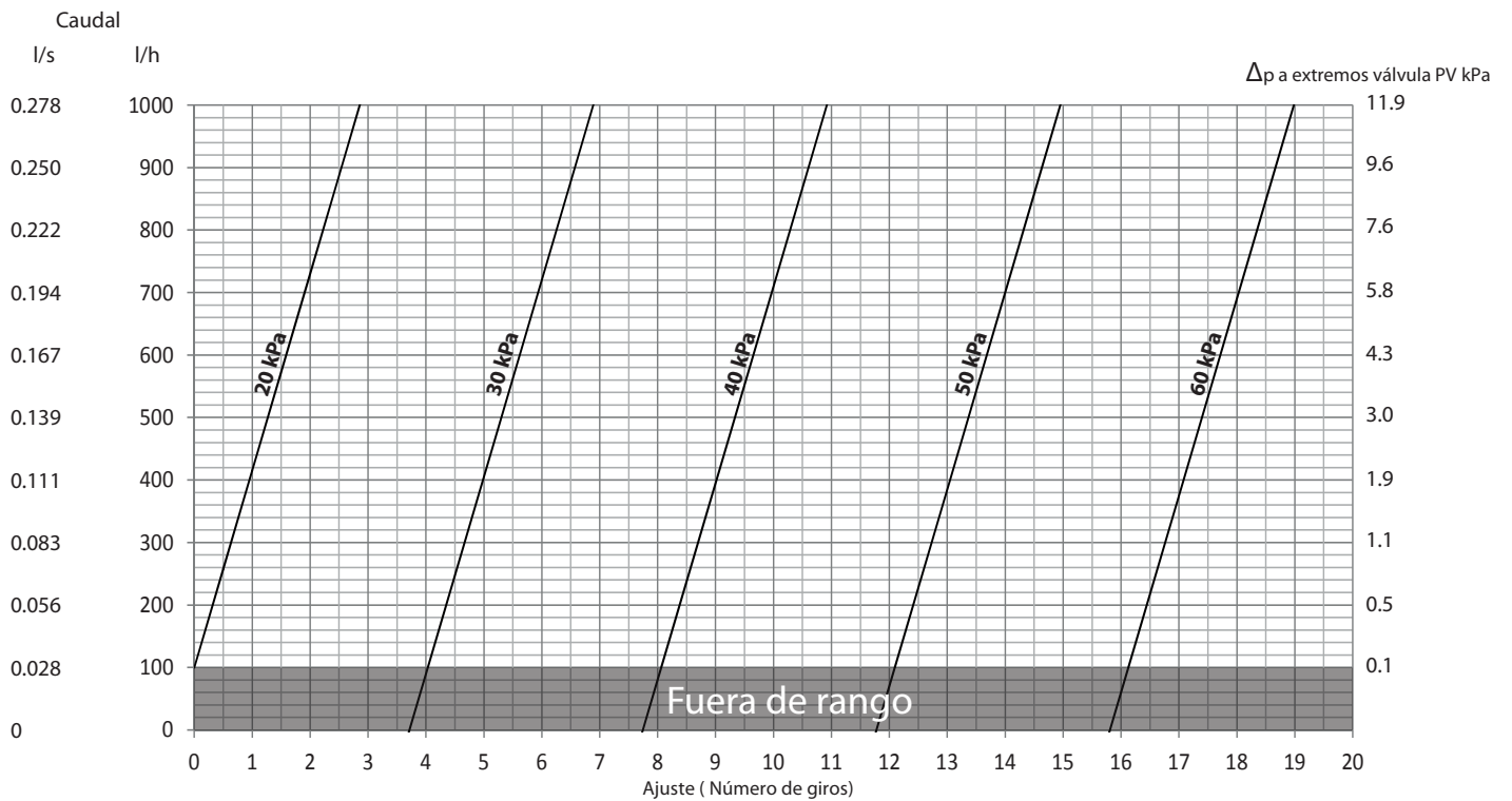
Gráfica de caudales Frese PV Compact DN 15, 20-60 kPa
