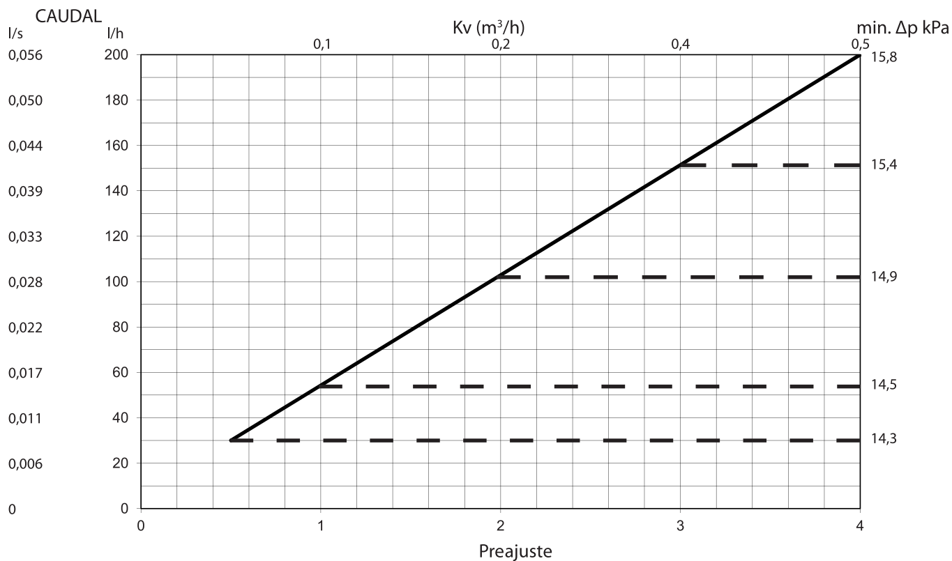
Gráfica de caudales Frese OPTIMA Compact DZR caudal bajo 5,0mm DN10/15
