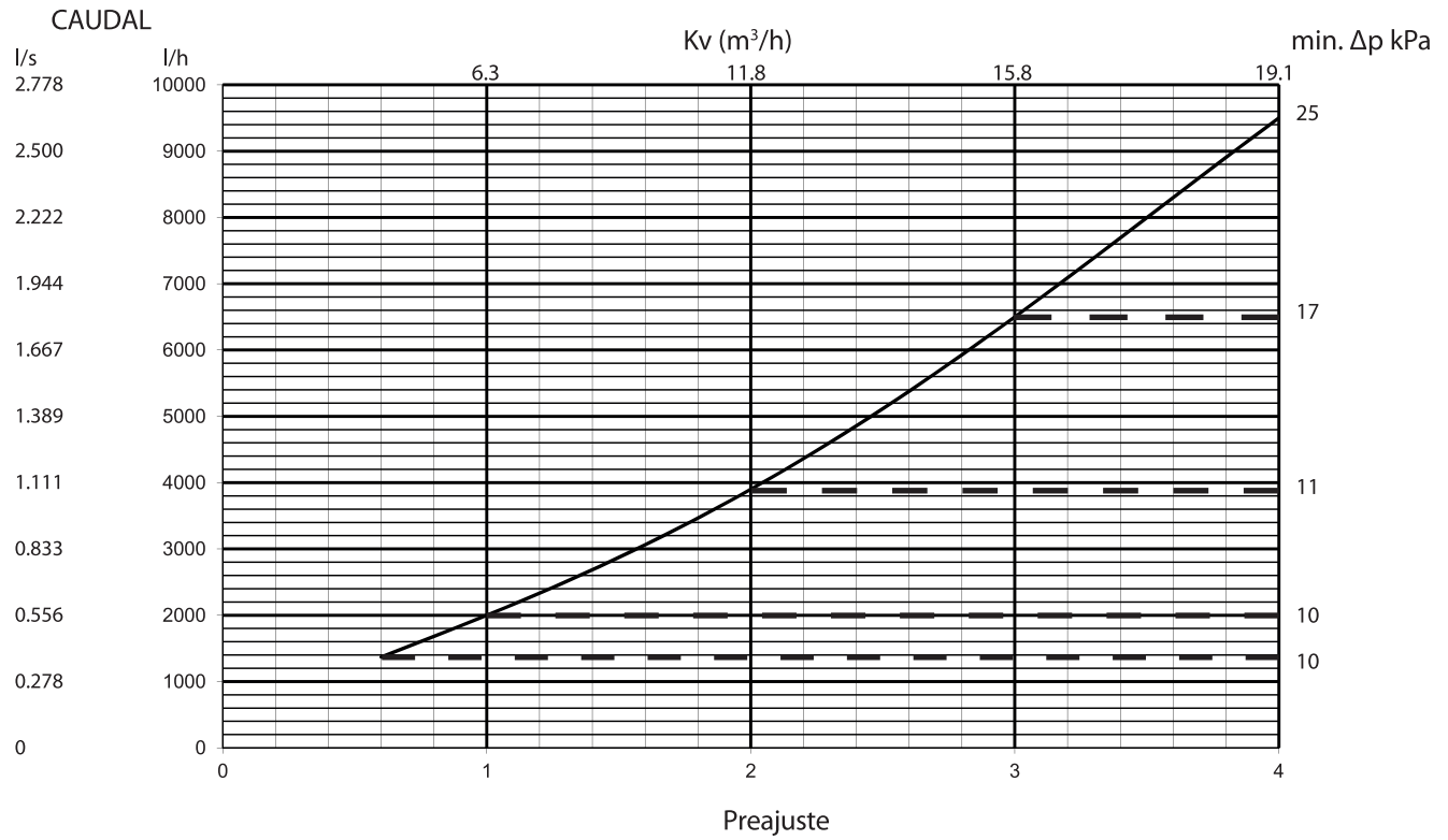
Gráfica de caudales Frese OPTIMA Compact DZR DN50
