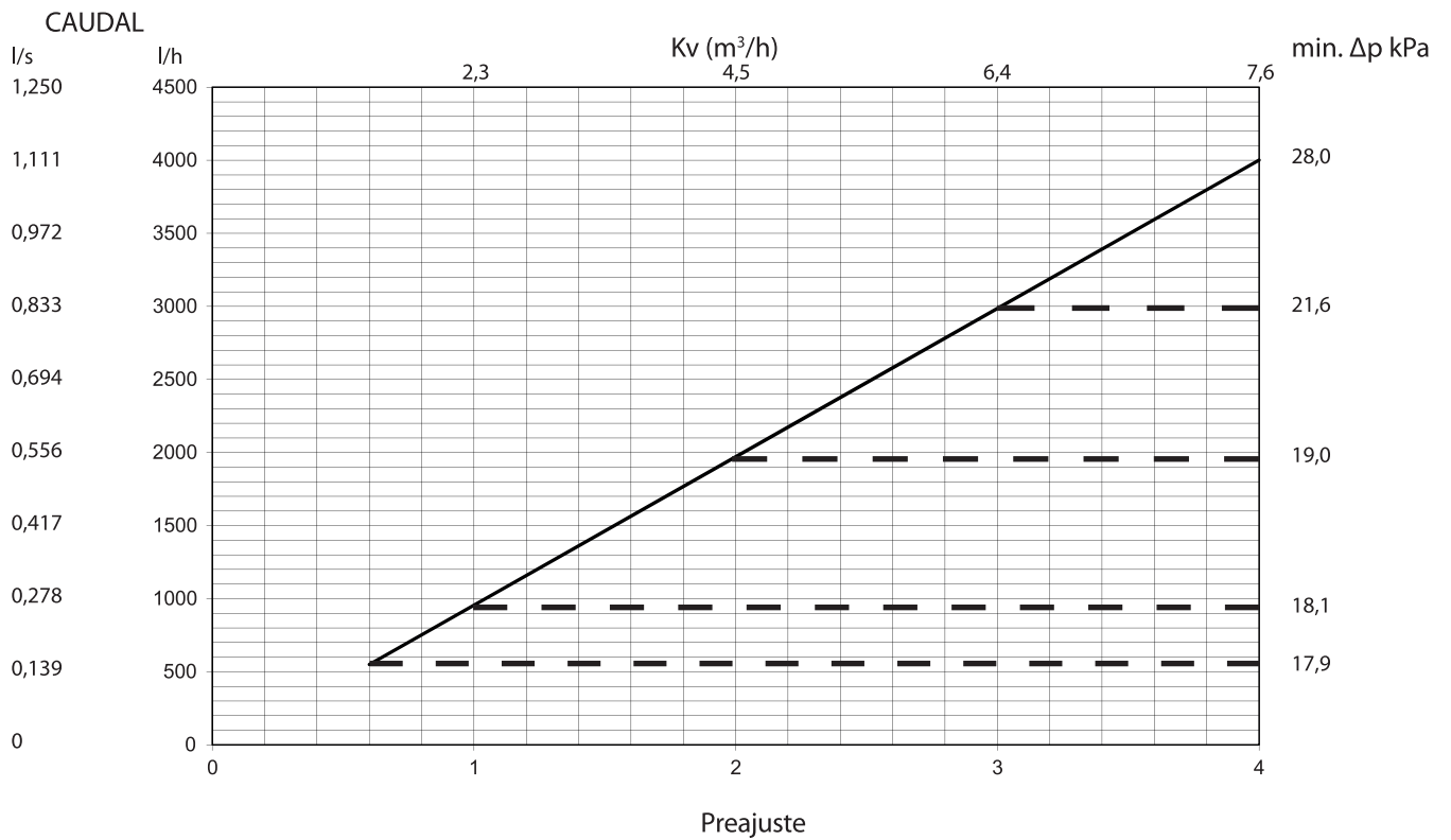
Gráfica de caudales Frese OPTIMA Compact DZR 5,5mm DN32
