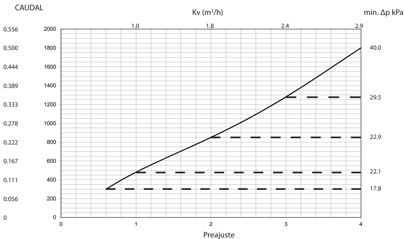
Gráfica de caudales Frese OPTIMA Compact DZR caudal bajo 5,5mm DN25
