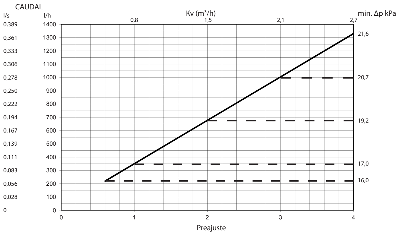
Gráfica de caudales Frese OPTIMA Compact DZR caudal alto 5,0mm DN15/20
